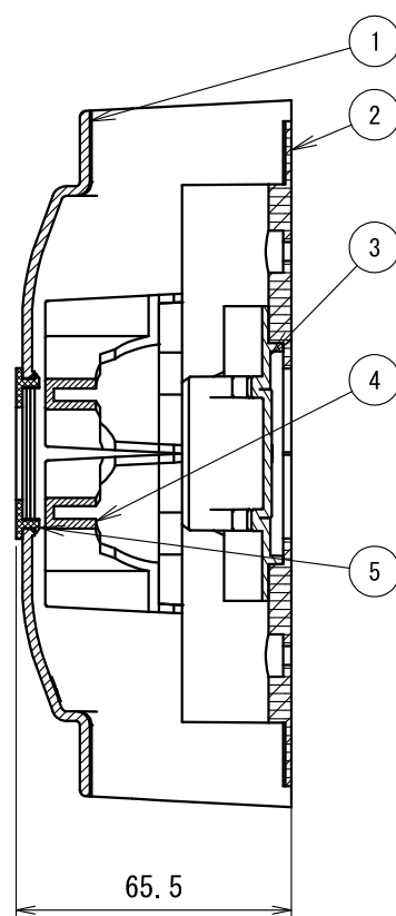
断面 A-A
